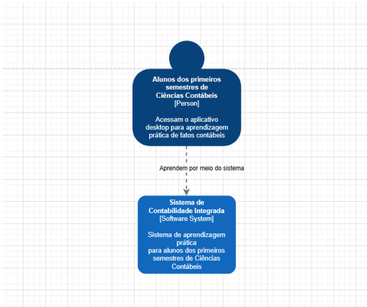
Diagrama C4 - Contexto
